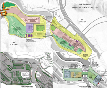
香港皇崗口岸 GROUND MASTER PLAN
